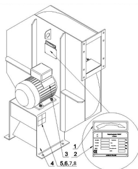
Napęd bezpośredni
