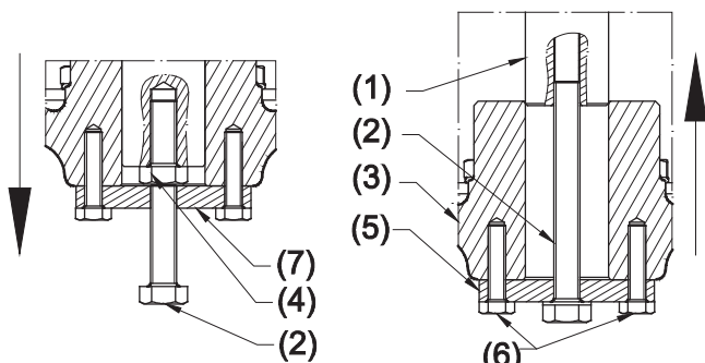
Demontaż wirnika
